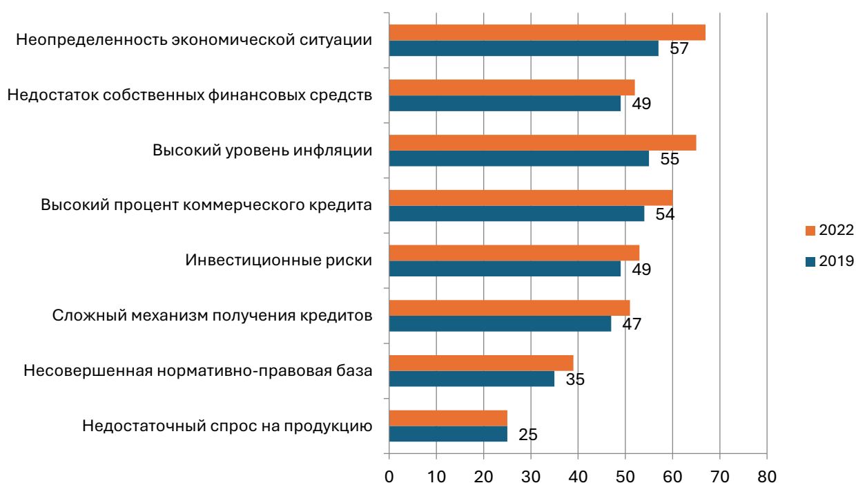
Рисунок 2. Распределение малых и средних предприятий по оценке проблем, ограничивающих инвестиционную деятельность в Российской Федерации за 2019-2022 гг., % [1], [2], [3]
