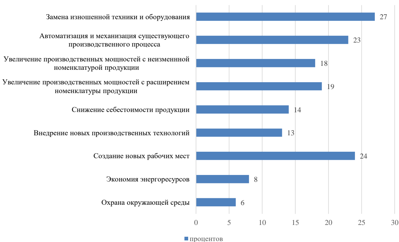
Рисунок 1. Распределение малых и средних предприятий по оценке целей инвестирования в основной капитал в Российской Федерации в 2022 г. (в процентах от общего числа организаций) [1], [2], [3]
